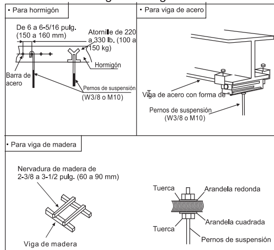
Fig. 3.2.1 Fijación de los pernos de suspensión
